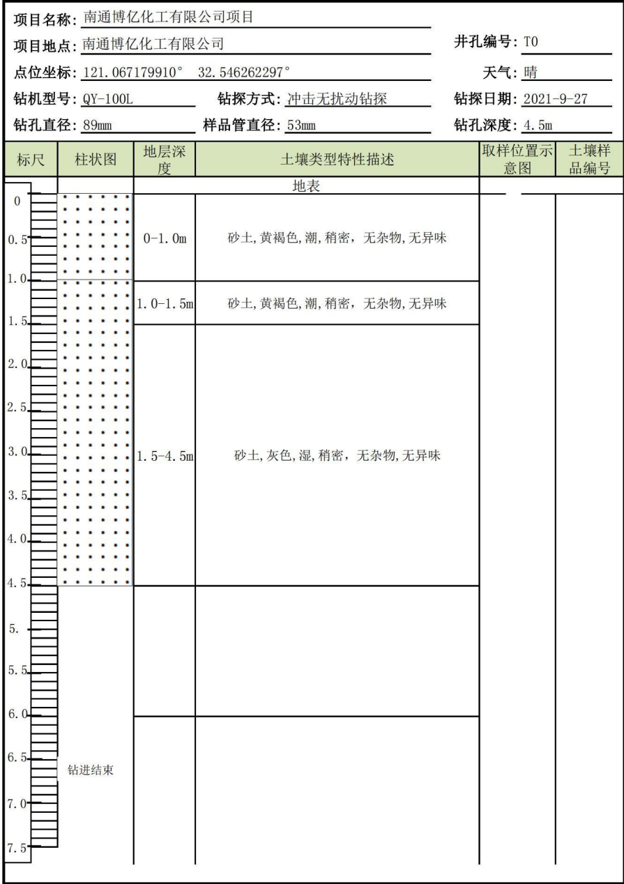
钻孔柱状图
