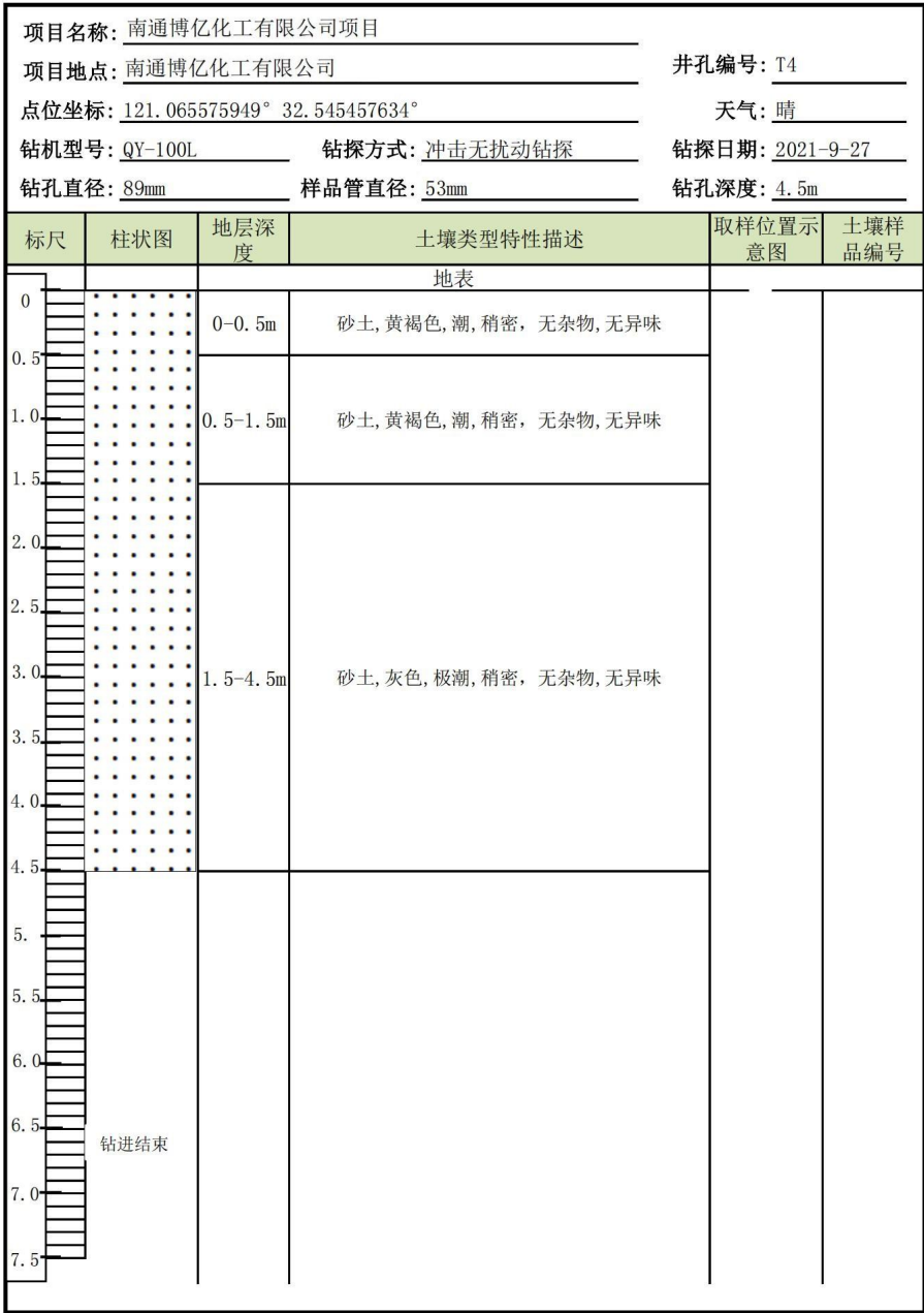
钻孔柱状图
